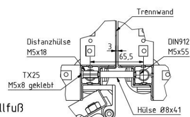
Detail A Anreihverbinder mit Trennwand
